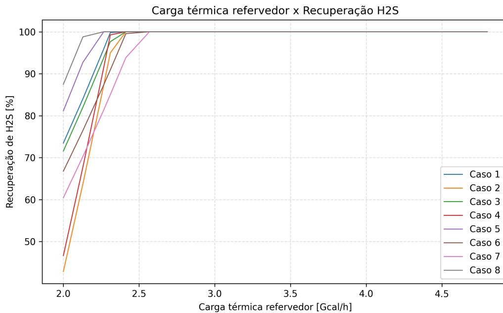
Figura 1: Carga térmica x recuperação de \text{H}_2\text{S}
