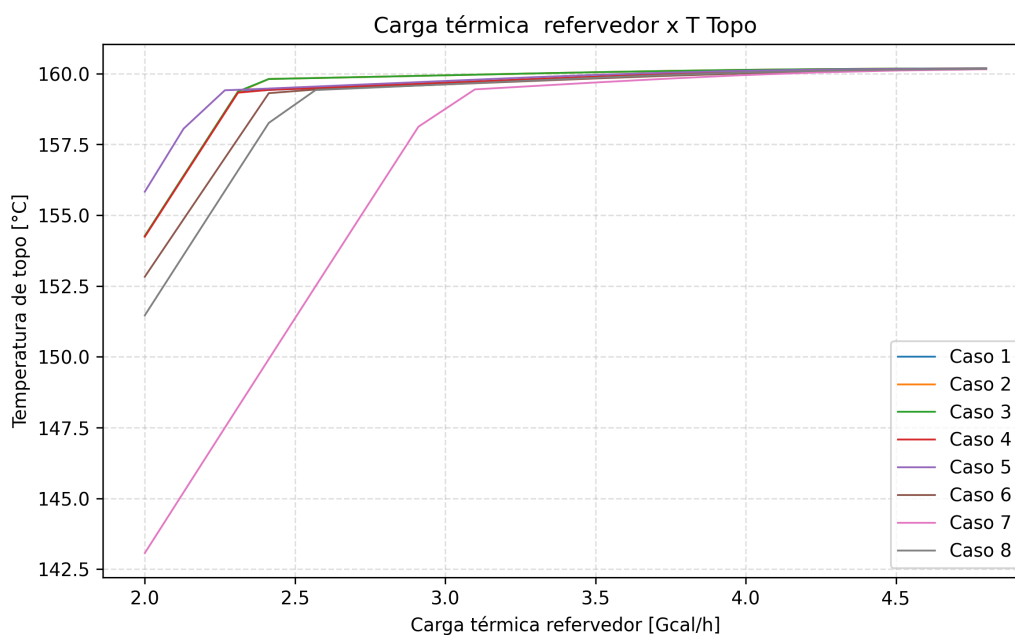
Figura 4: Carga térmica x temperatura do topo
