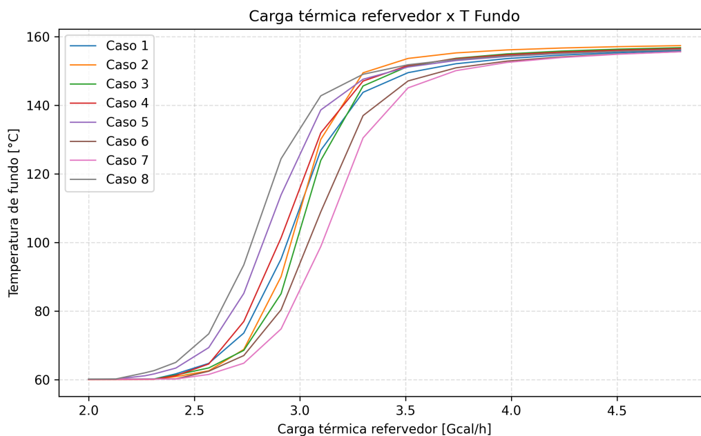
Figura 3: Carga térmica x temperatura do fundo
