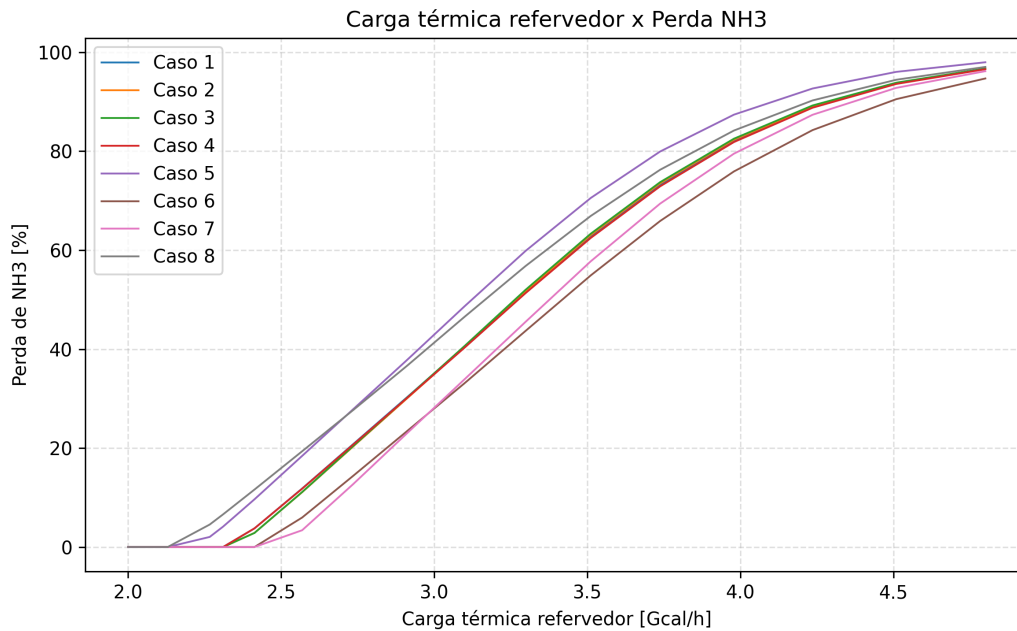
Figura 2: Carga térmica x perda de \text{NH}_3
